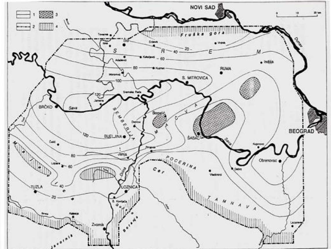
Slika 11. Karta temperature geotermalnih voda ( ^{\circ}\text{C} ) na gornjoj granici rezervoara od trijaskih krečnjaka (1-izoterma; 2-granica modela; 3-područje bez krečnjaka; 4-područje hladnih voda u rezervoaru)
